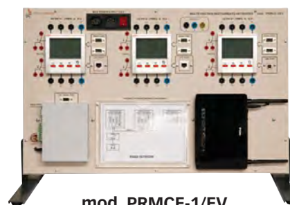
mod. PRMCE-1/EV Monitoraggio dei consumi di energia elettrica con reti SCADA
