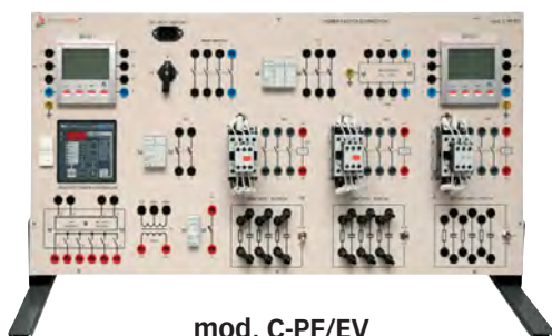
mod. C-PF/EV Impianti di rifasamento automatico
